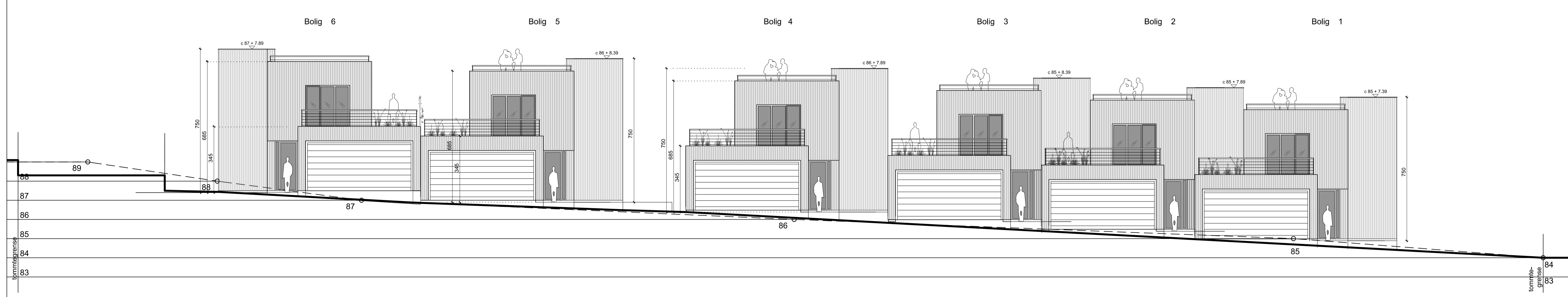
Østfasade Boliger 1-6
